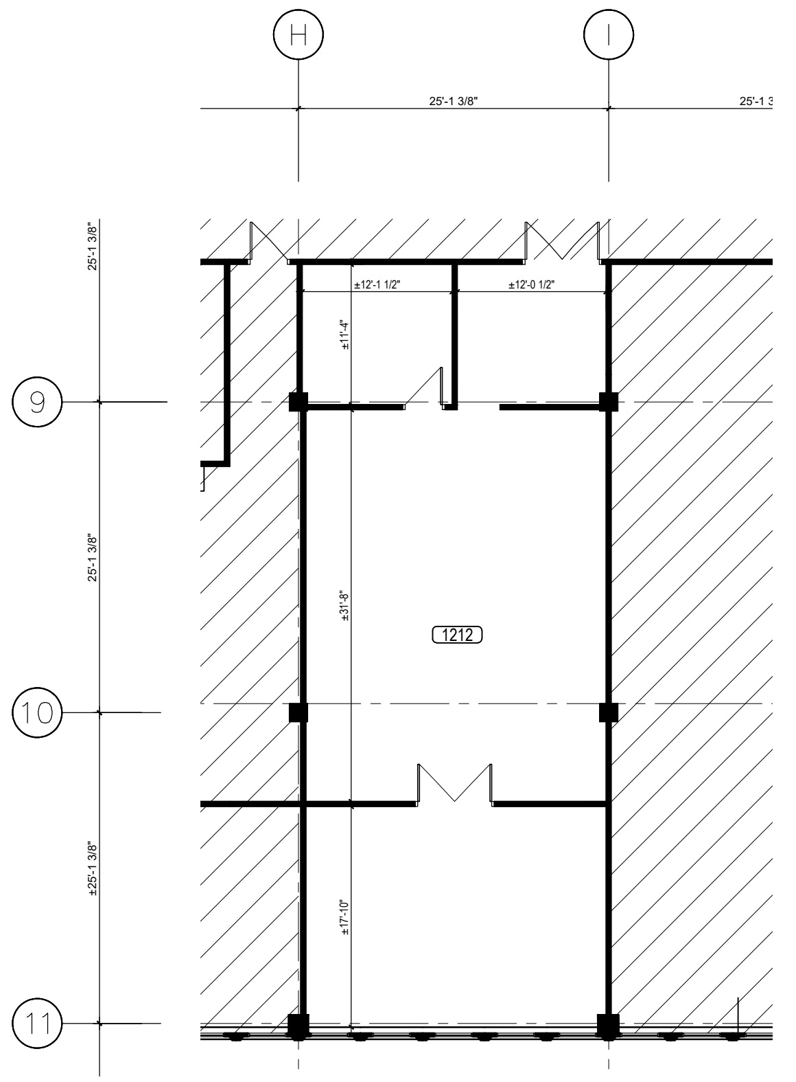
LOCAL 1212 PLAN DE LA SUITE 01 ÉCHELLE: 3/32" = 1'-0" A-01
